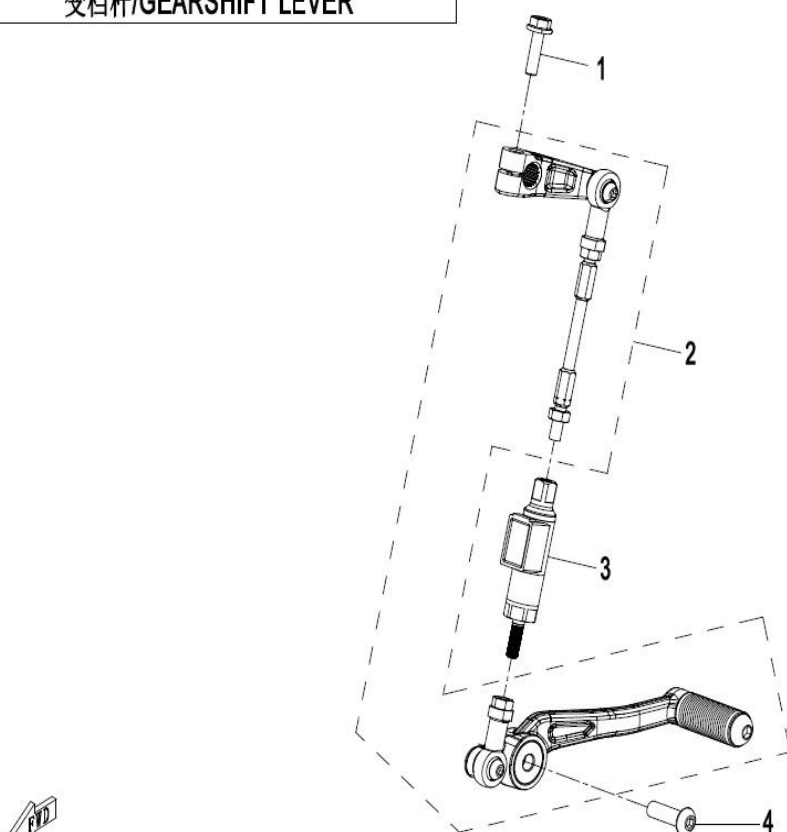
F14-2 GEARSHIFT LEVER
