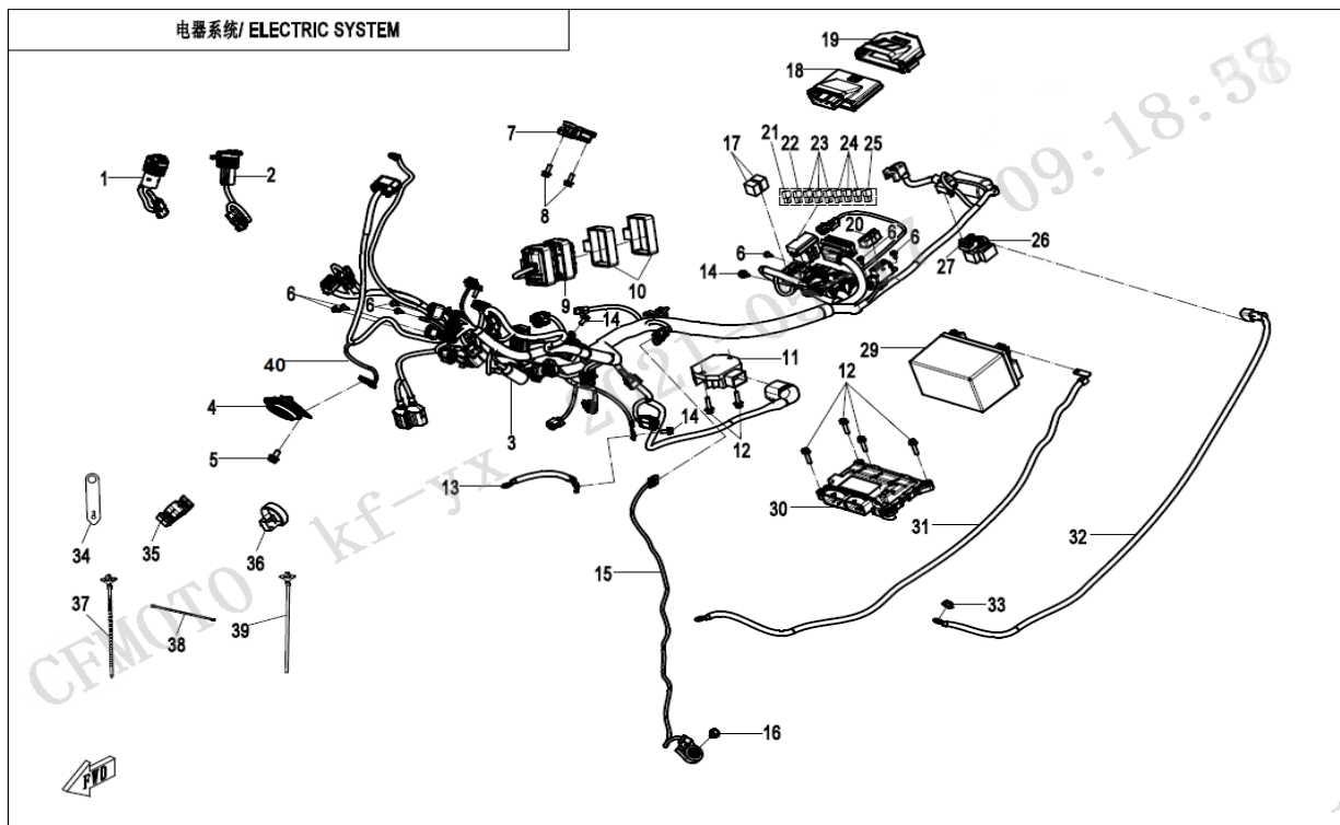
F15-1-A ELECTRIC SYSTEM(SPORT)
